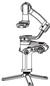
Состояние блокировки для установки камеры
