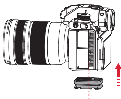
Состояние блокировки для установки камеры
